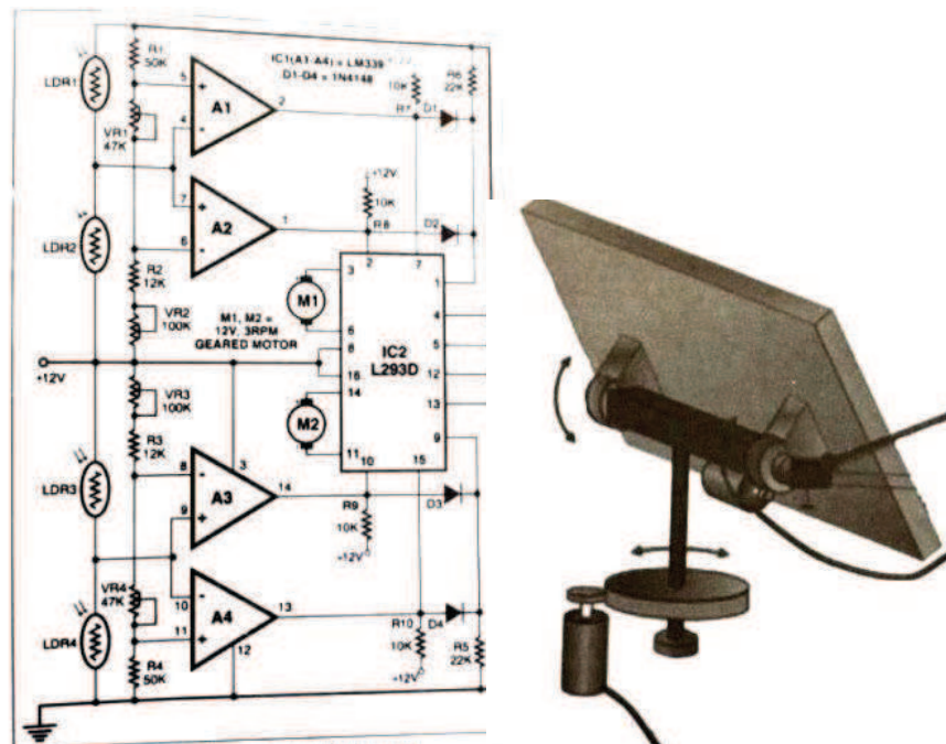
Gambar 3.3 Rangkaian elektronik sistem pelacakan surya
