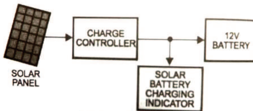
Gambar 3.5 Blok diagram indikator pengisian baterai tenaga surya
